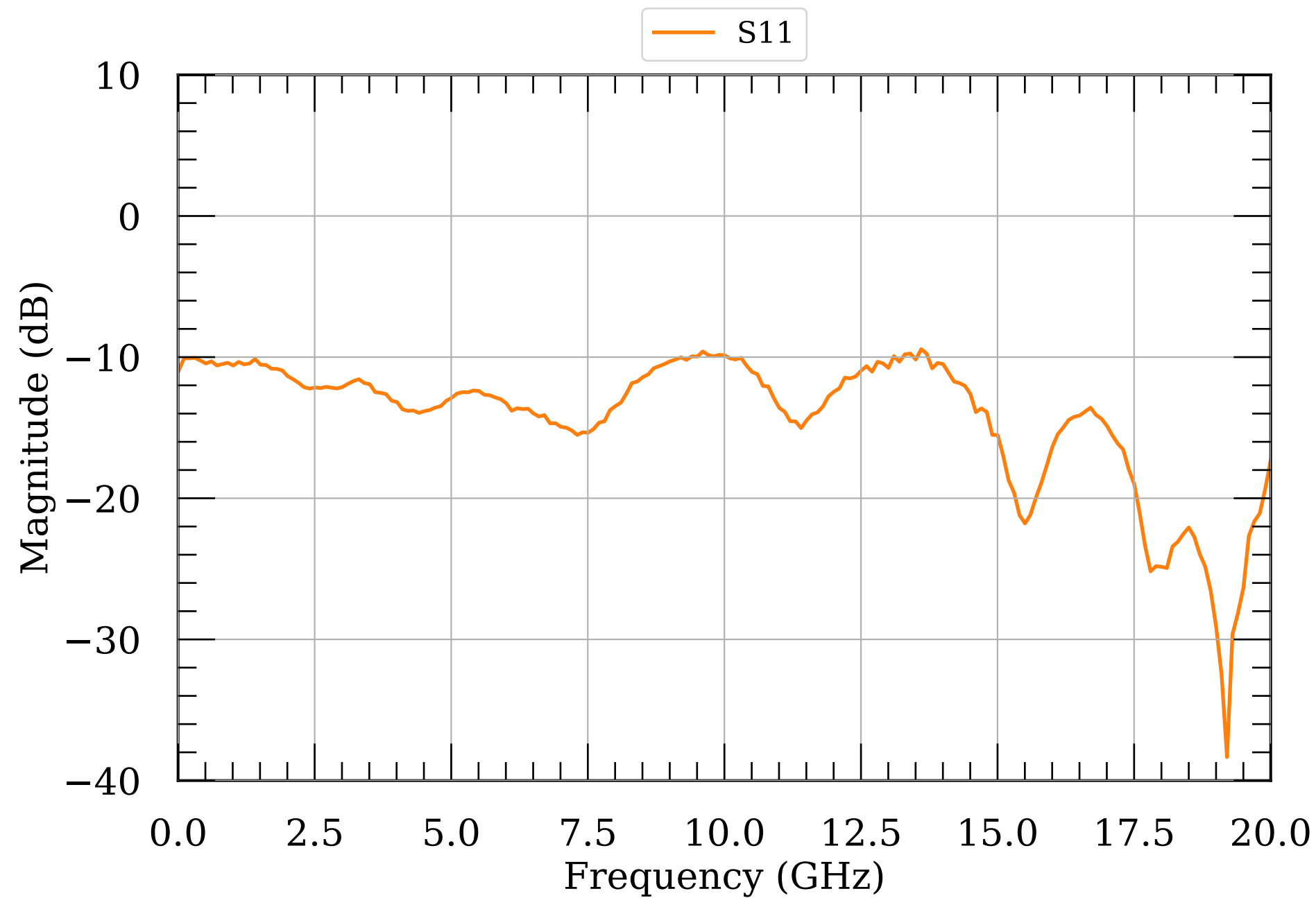
LNA S-params module011
